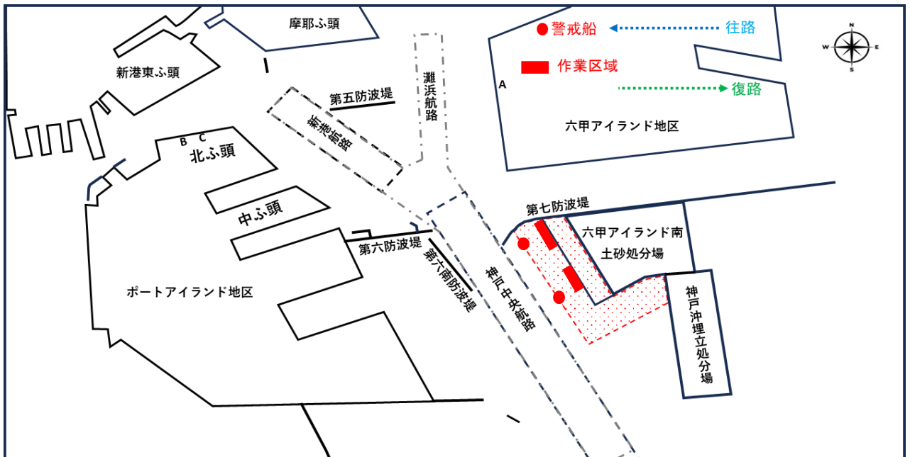
(工事作業位置・運搬経路等略図)
